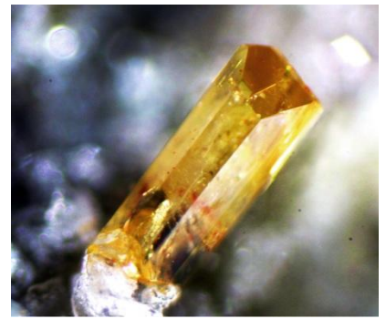
Monazite
