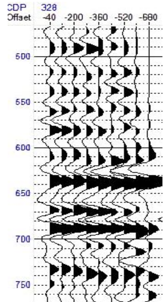
Actual Synthetic seismogram
