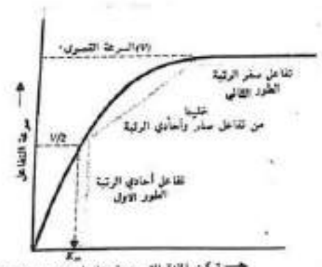
تؤثر تركيز المادة التي يعمل عليها الأيون (المادة المتفاعلة) على سرعة التفاعل . بالتزامن مع تركيز الأيون المتفاعل.
