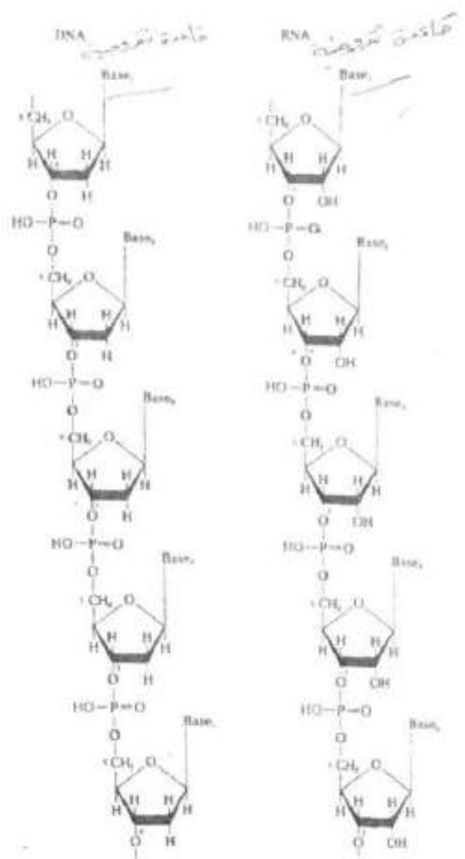
شكل (4-6) تركيب النيوكليوتيدات المتعددة في DNA و RNA ، لاحظ ان الارتباط بين جزيئي نيوكليوتيد يكون بواسطة جسر فوسفاتي على الآسرة التي بين مجموعة الفسفرات - 2 نيوكليوتيد ومجموعة الفسفرات - 3 نيوكليوتيد التي
