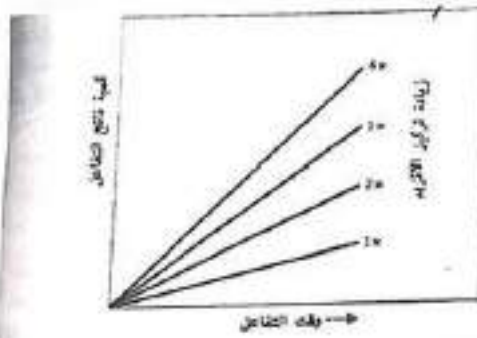
يؤثر تركيز الأيون على سرعة التفاعل ، بالتزامن مع وجود مادة من المادة التي يعمل عليها الأيون وللمادة المتفاعلة.
