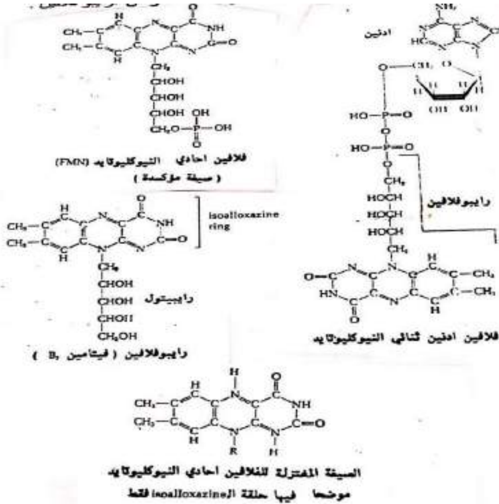
شكل (١٠ - ١) الرايبوفلافين واشكاله من مراقبات الانهم
