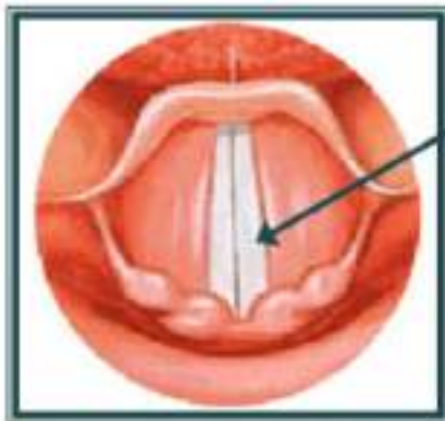
حالة الجهر
