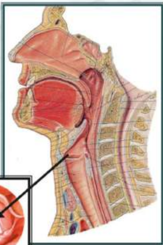
الوترين الصوتيين
