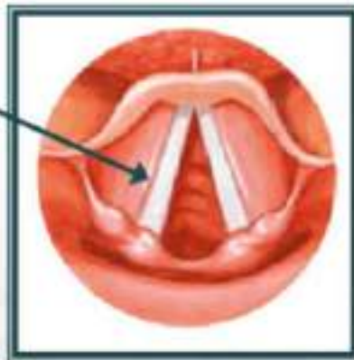
حالة الهمس
