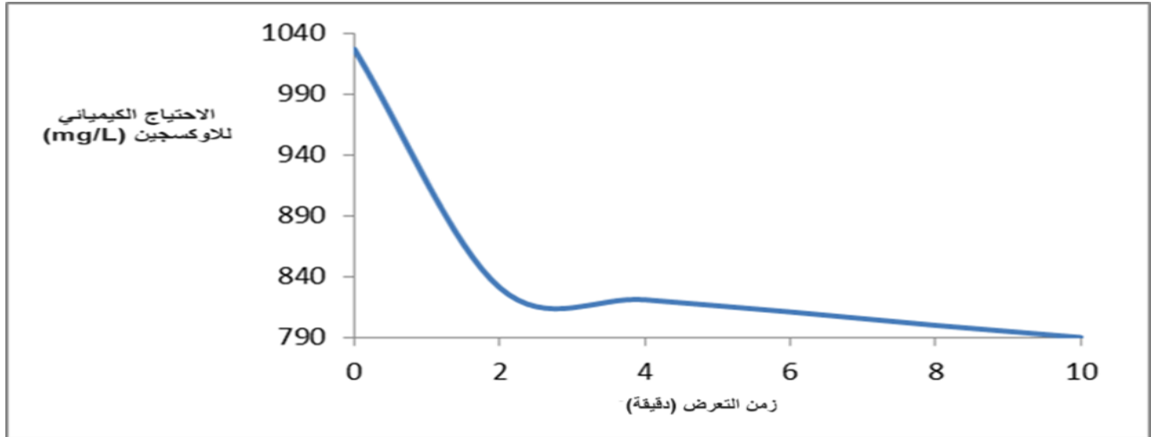
شكل (3): العلاقة بين الاحتياج الكيميائي للأوكسجين وزمن التعرض للأمواج فوق الصوتية
