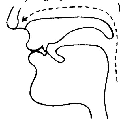
Fig. 20 /m/
